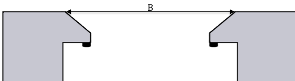
Pasvirusio lango rėmo pjūvio vaizdas iš viršaus
