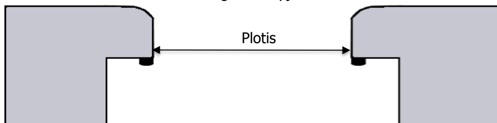
Standartinio lango rėmo pjūvio vaizdas iš viršaus
